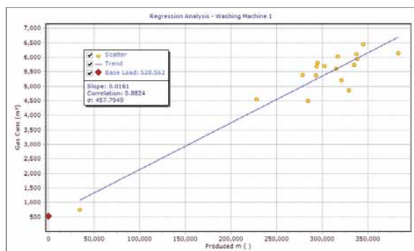
Fig. 7: Linha Característica de Performance (PCL).
