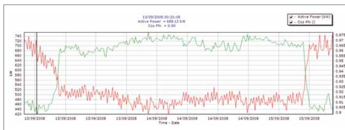
Fig. 2: Relatório de contagem do contador principal da fábrica. O consumo de electricidade (potência activa) e o respectivo factor de potência (cos phi) são registados em intervalos de 15 minutos. Durante o fim-de-semana apenas algumas máquinas estão a produzir e como resultado a potência activa diminui e o factor de potência melhora. O gráfico mostra que o factor de potência permanece sempre acima de 0,9, o que indica uma situação aceitável. Este gráfico também permite avaliar o funcionamento das baterias de condensadores para melhorar o factor de potência.
