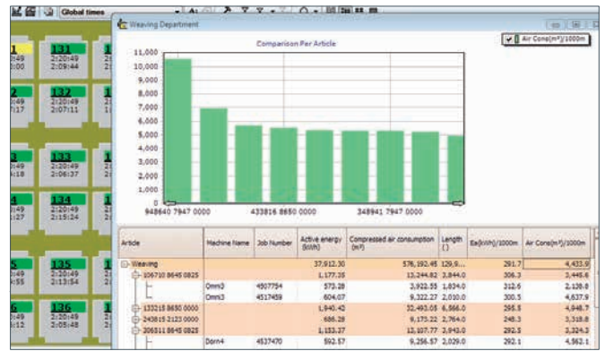
Vista de la planta con el informe del ENERGYMASTER (comparación del consumo energético por artículo).
