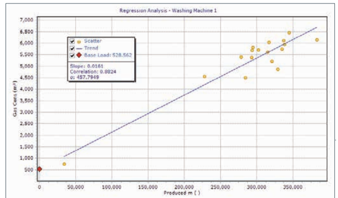
Performance Characteristic Line (PCL) para el consumo de gas de una línea de lavado.
