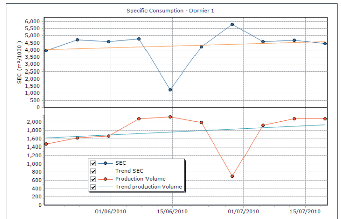
Evolución del Specific Energy Consumption (SEC), aire de un telar Dornier.
