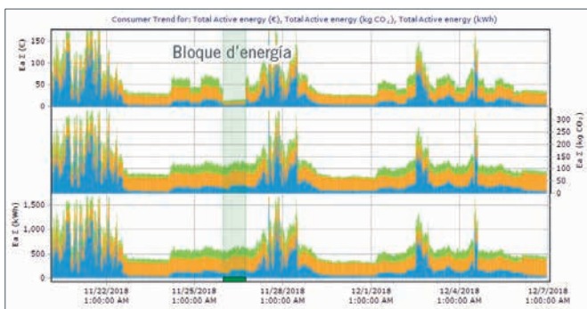
Consumo emisiones CO 2 y coste de tres consumidores.
